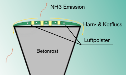
Die spezielle Form sorgt für geringere Ammoniakemissionen und einen angenehmen Untergrund
