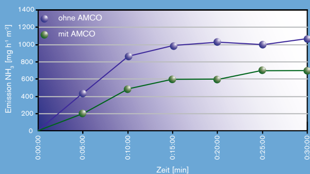
Messung der Ammoniakwerte im Zeitverlauf 1
